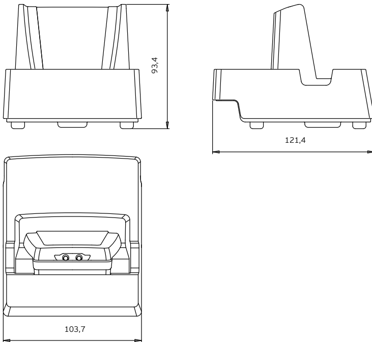
Abb. 13: Ladestation (Maße in Millimetern)
